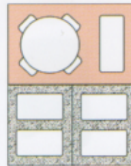
6. KOMÍNOVÁ TVÁRNICE 35x50 CM + 2x VENTILAČNÍ TVÁRNICE 35x25 CM
